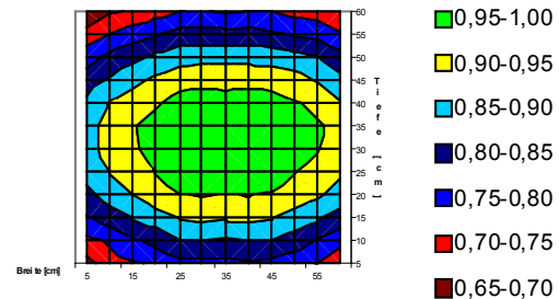
Abb. 2: Bestrahlungsstärke auf der Grundfläche
