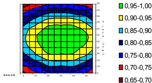
Abb. 2: Bestrahlungsstärke auf der Grundfläche
